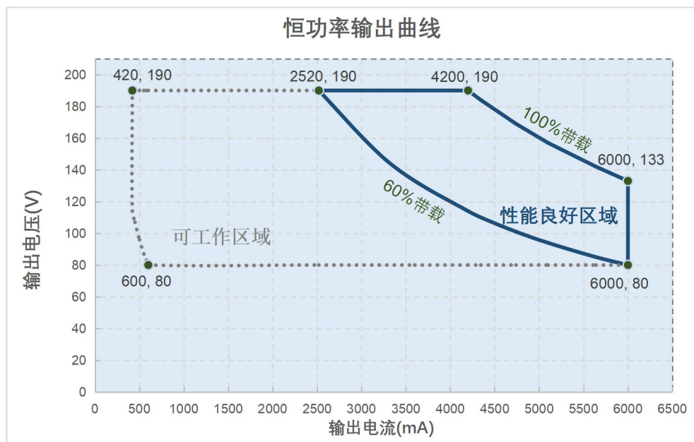
EBB-800-6A00-N Model 工作曲线图
