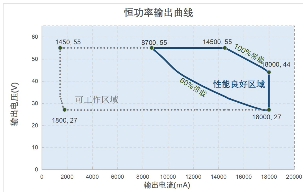
EBB-800-18A0-N Model 工作曲线图
