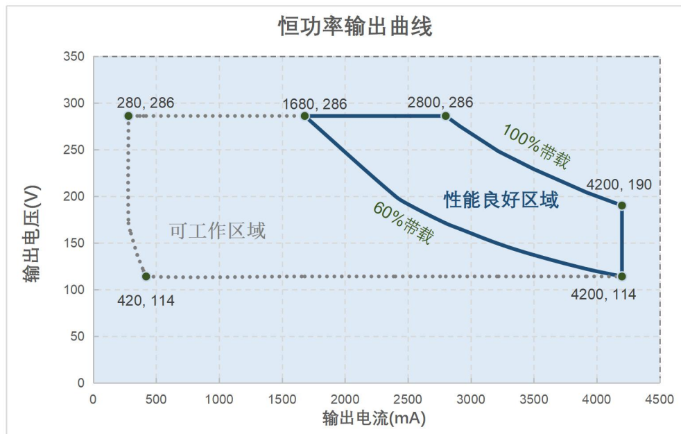
EBB-800-4A20-N Model 工作曲线图
