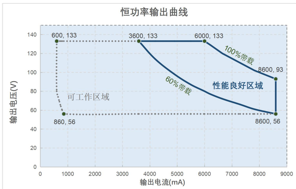
EBB-800-8A60-N Model 工作曲线图
