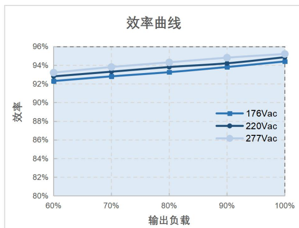
EBB-800-18A0-D Model 工作曲线
