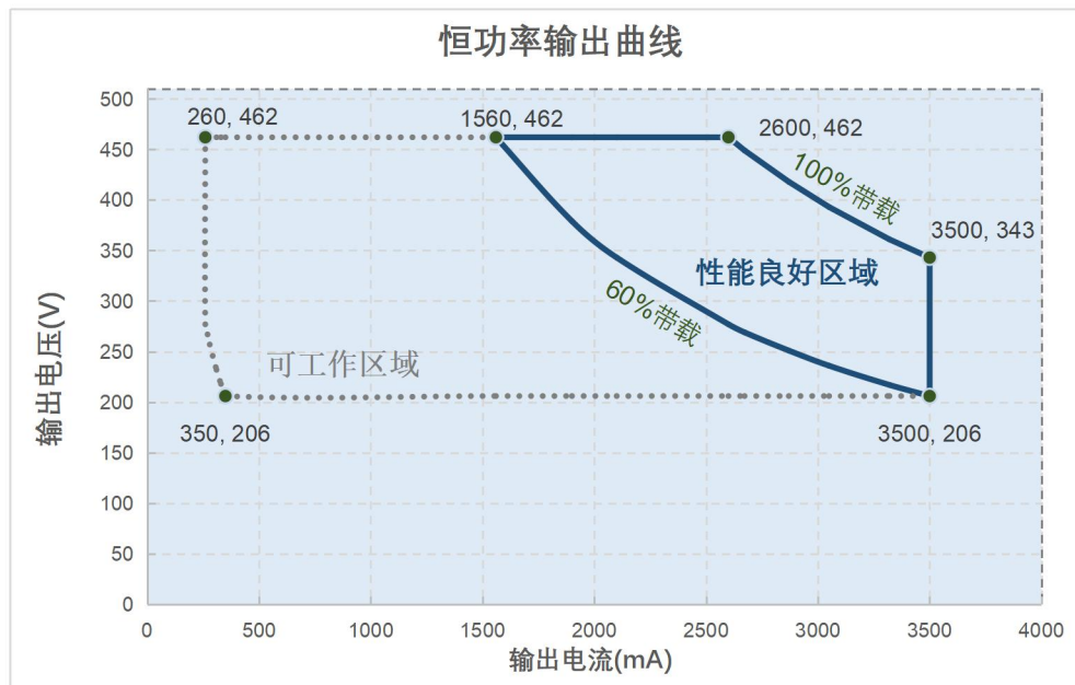
EBB-1K2-3A50-D Model 工作曲线图
