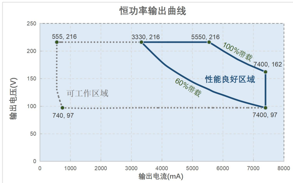
EBB-1K2-7A40-D Model 工作曲线图
