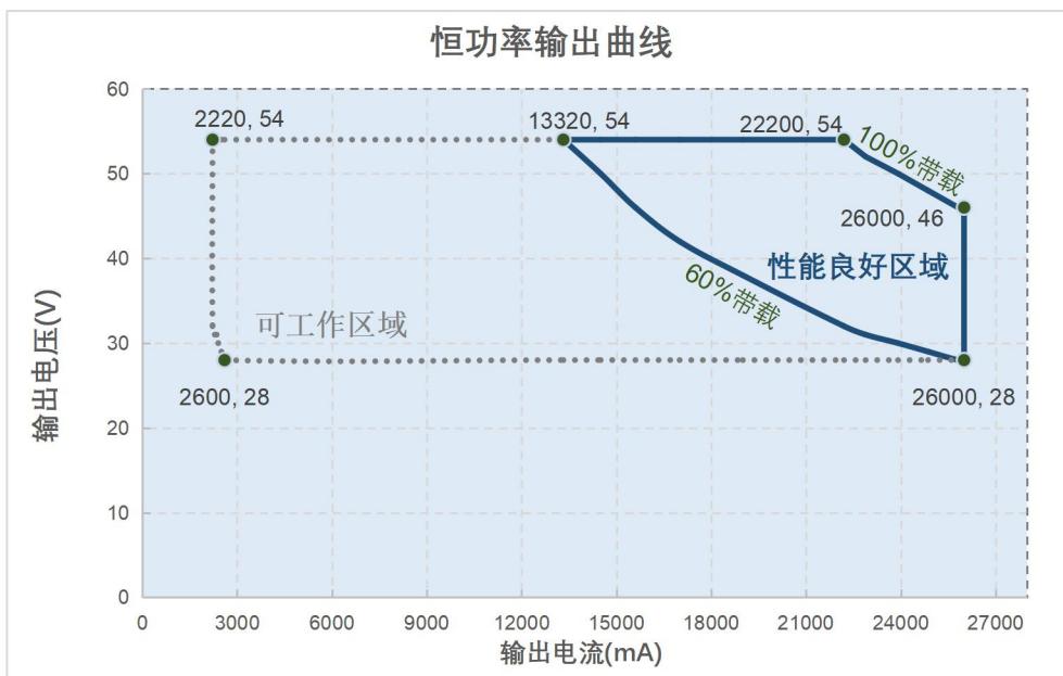
EBB-1K2-26A0-D Model 工作曲线图
