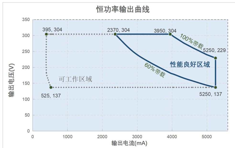
EBB-1K2-5A25-D Model 工作曲线图
