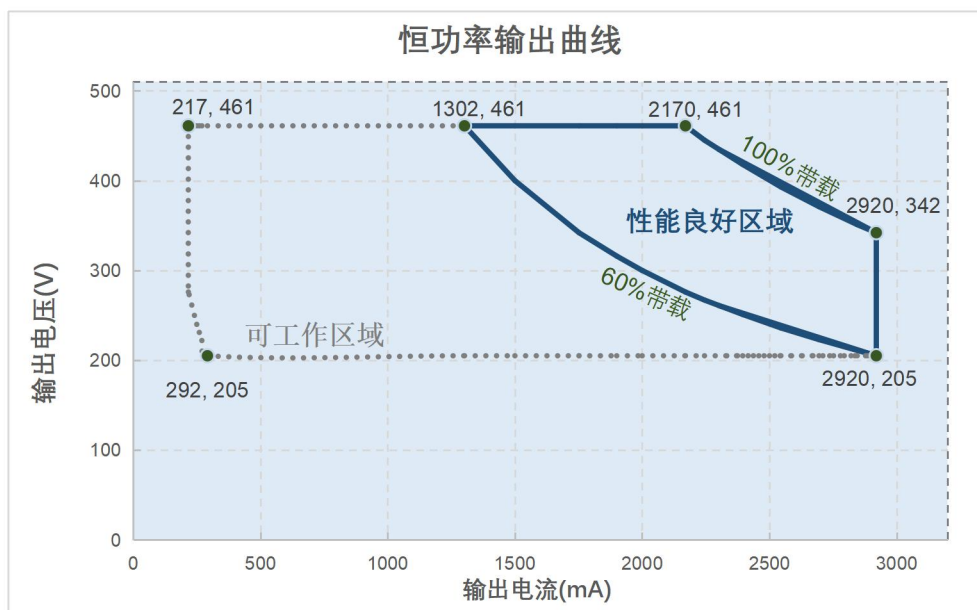
EBB-1K0-2A92-N Model 工作曲线图
