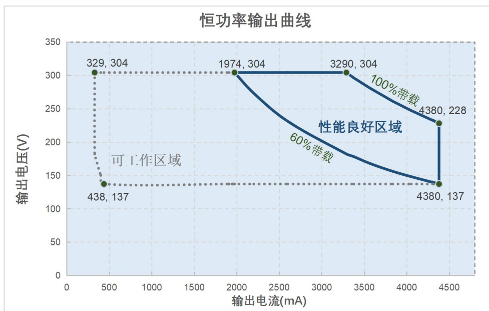
EBB-1K0-4A38-N Model 工作曲线图
