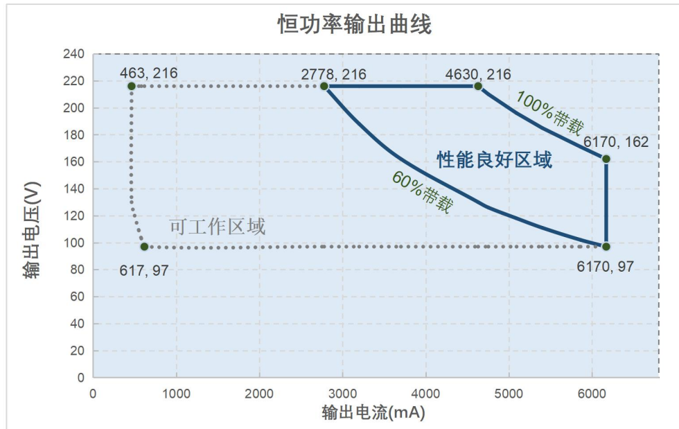
EBB-1K0-6A17-N Model 工作曲线图
