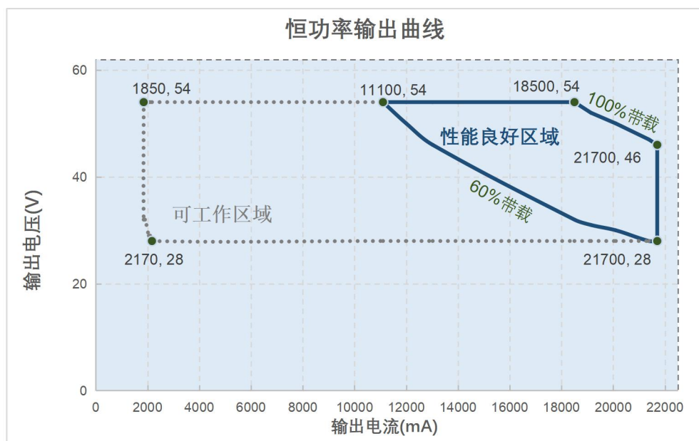
EBB-1K0-21A7-N Model 工作曲线图
