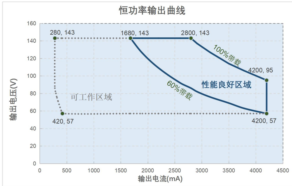
EBB-400-4A20-N Model 工作曲线图
