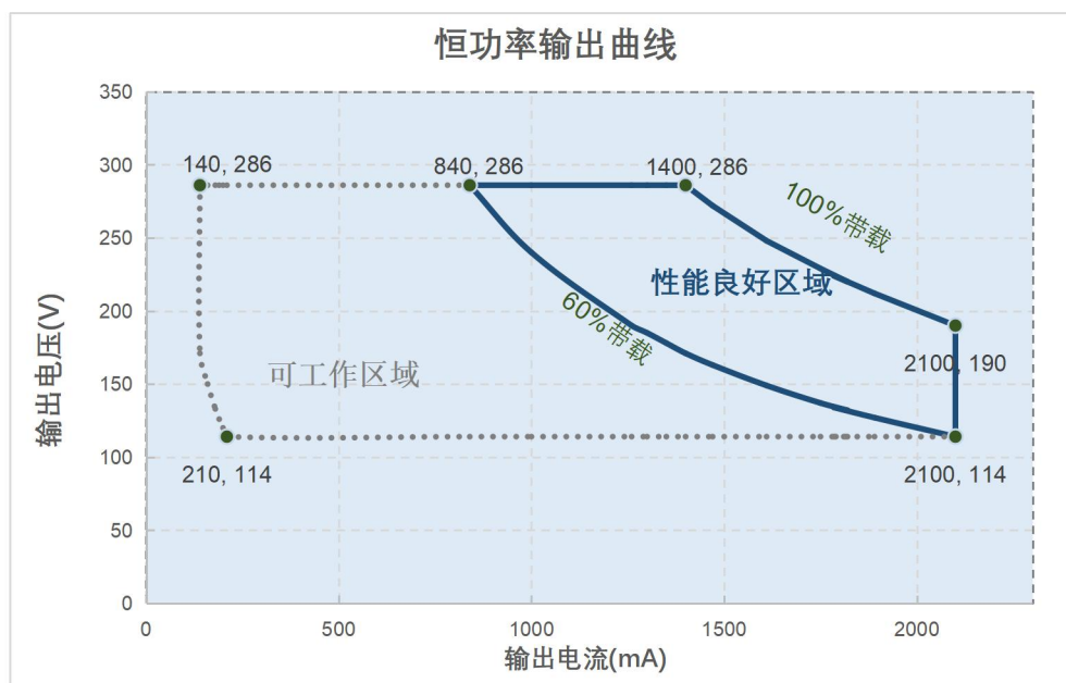
EBB-400-2A10-N Model 工作曲线图
