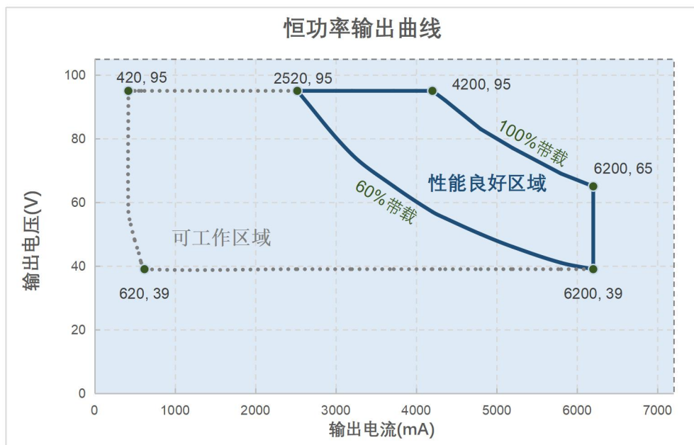
EBB-400-6A20-N Model 工作曲线图
